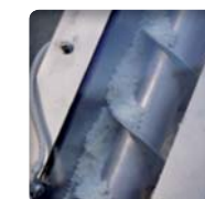
Capots de l'auge implantés sur les charnières avec gâche de sécurité pour accéder facilement à l'intérieur de l'auge ou surface en plexiglas
