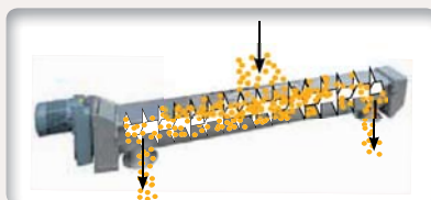
Exemple de vis à deux sens de marche 1 entrée rectangulaire centrale avec 2 sorties rondes opposées.
