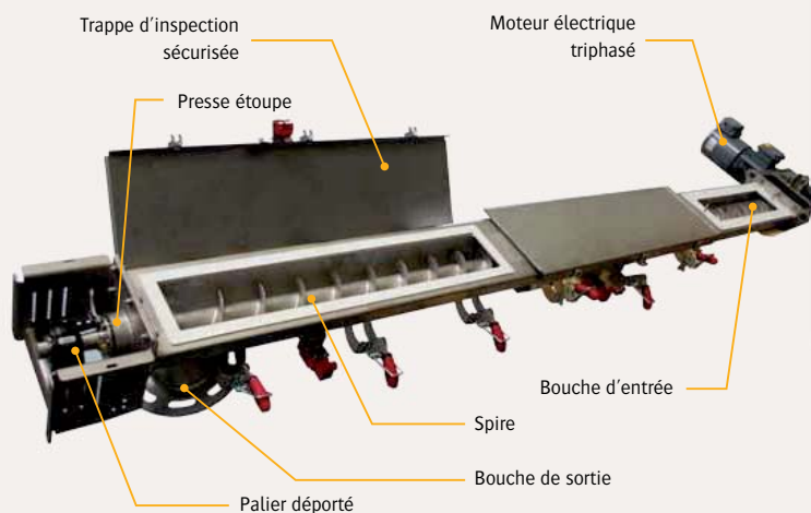
Auges multi-bouches pour alimenter plusieurs points de réception du produit
